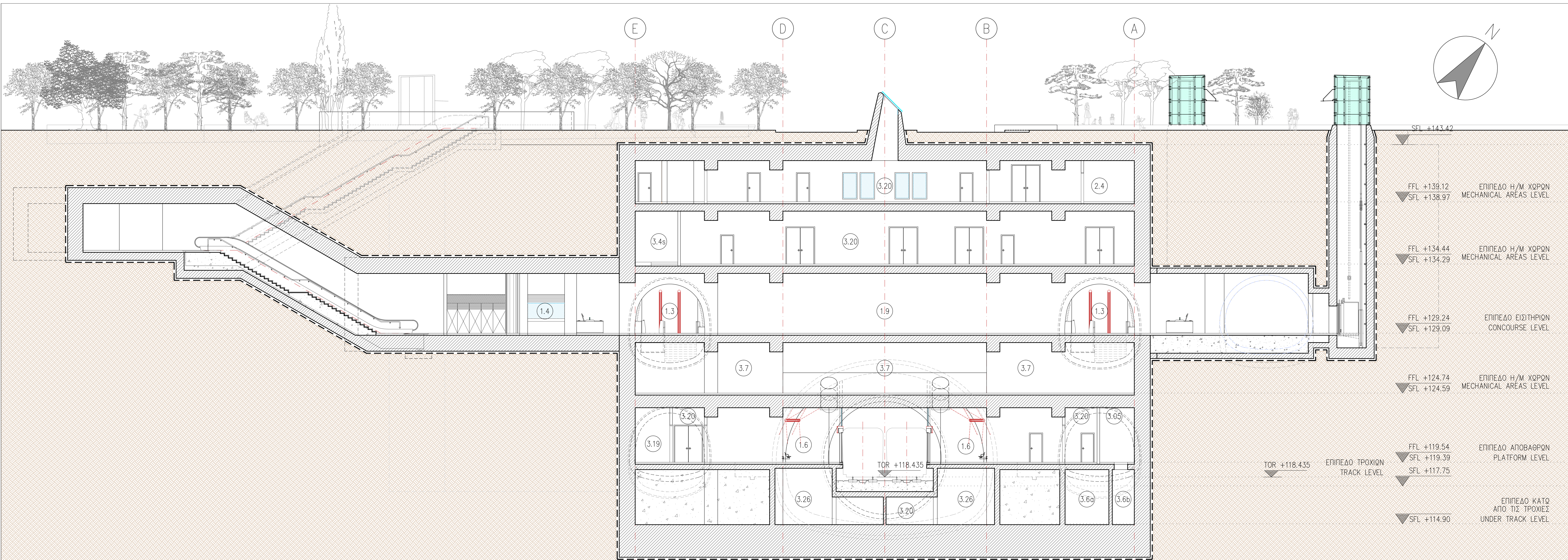
TOMH B-B
