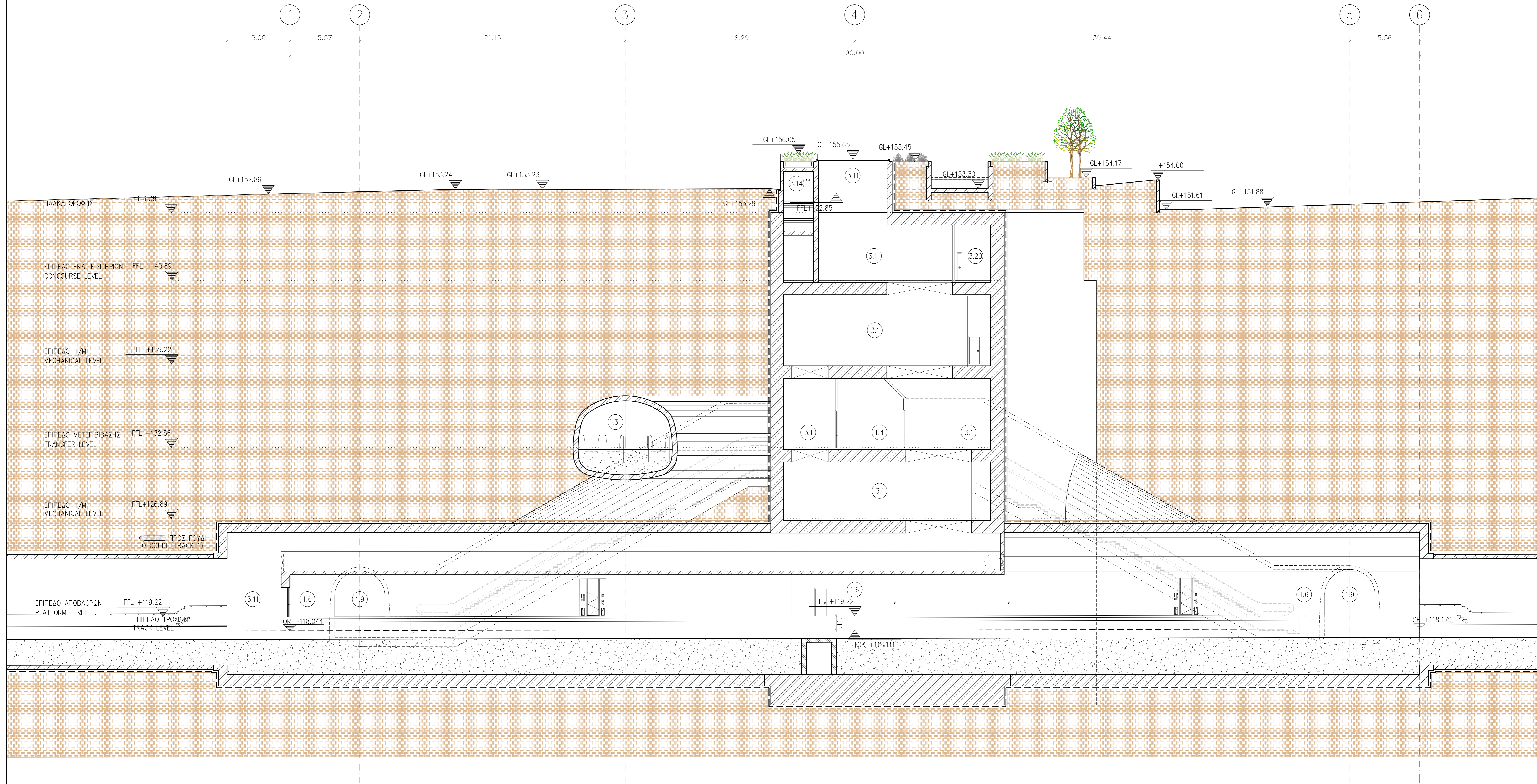
ΤΟΜΗ Α-Α ΚΑΙΜΑΚΑ 1:200
