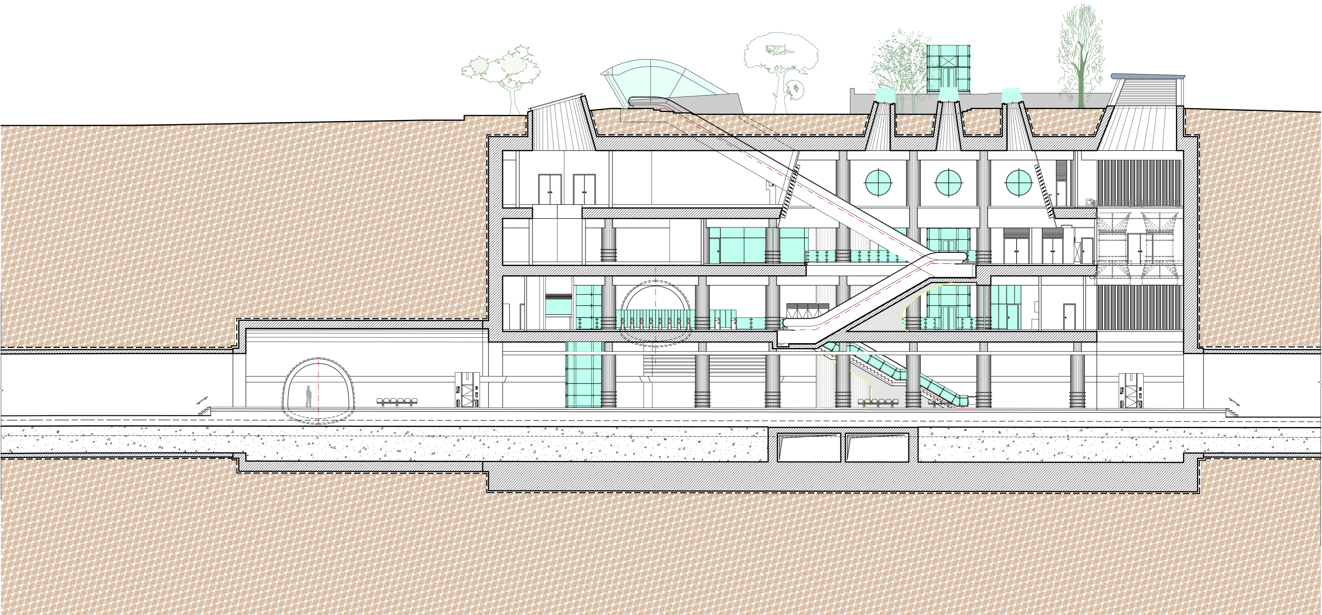
TOMH A-A
