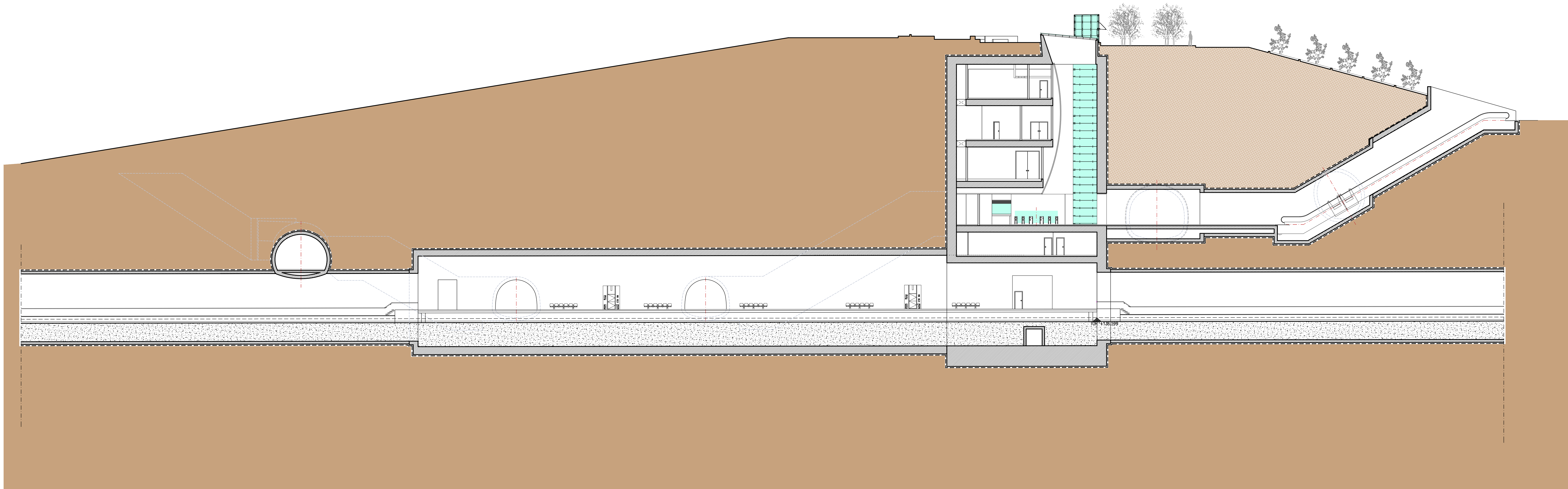
TOMH A-A
